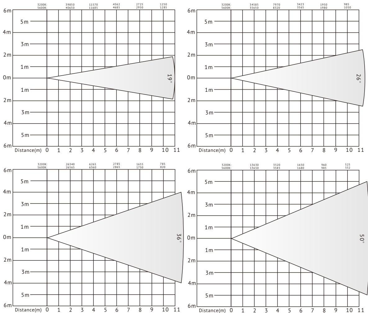
Lux Chart of VanGaa ERS200A
